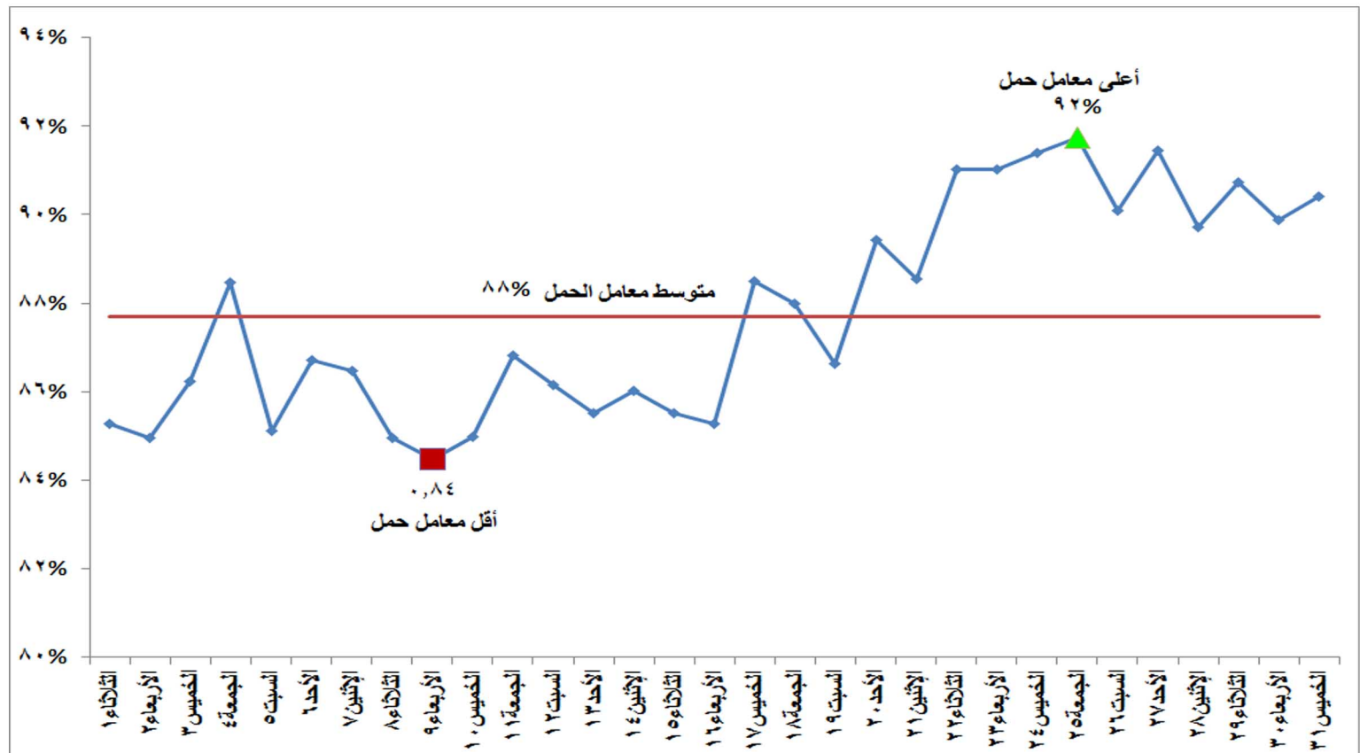
شكل (١٢) إجمالي معامل الحمل لوحدات الانتاج خلال شهر مايو ٢٠١٨
