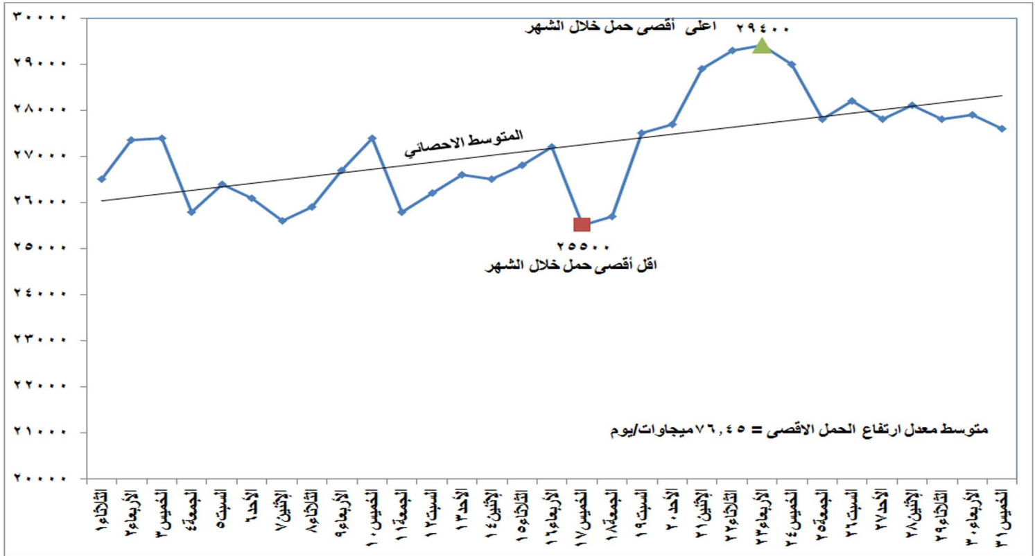
شكل (١) تطور الحمل الاقصى اليومي خلال شهر مايو ٢٠١٨
