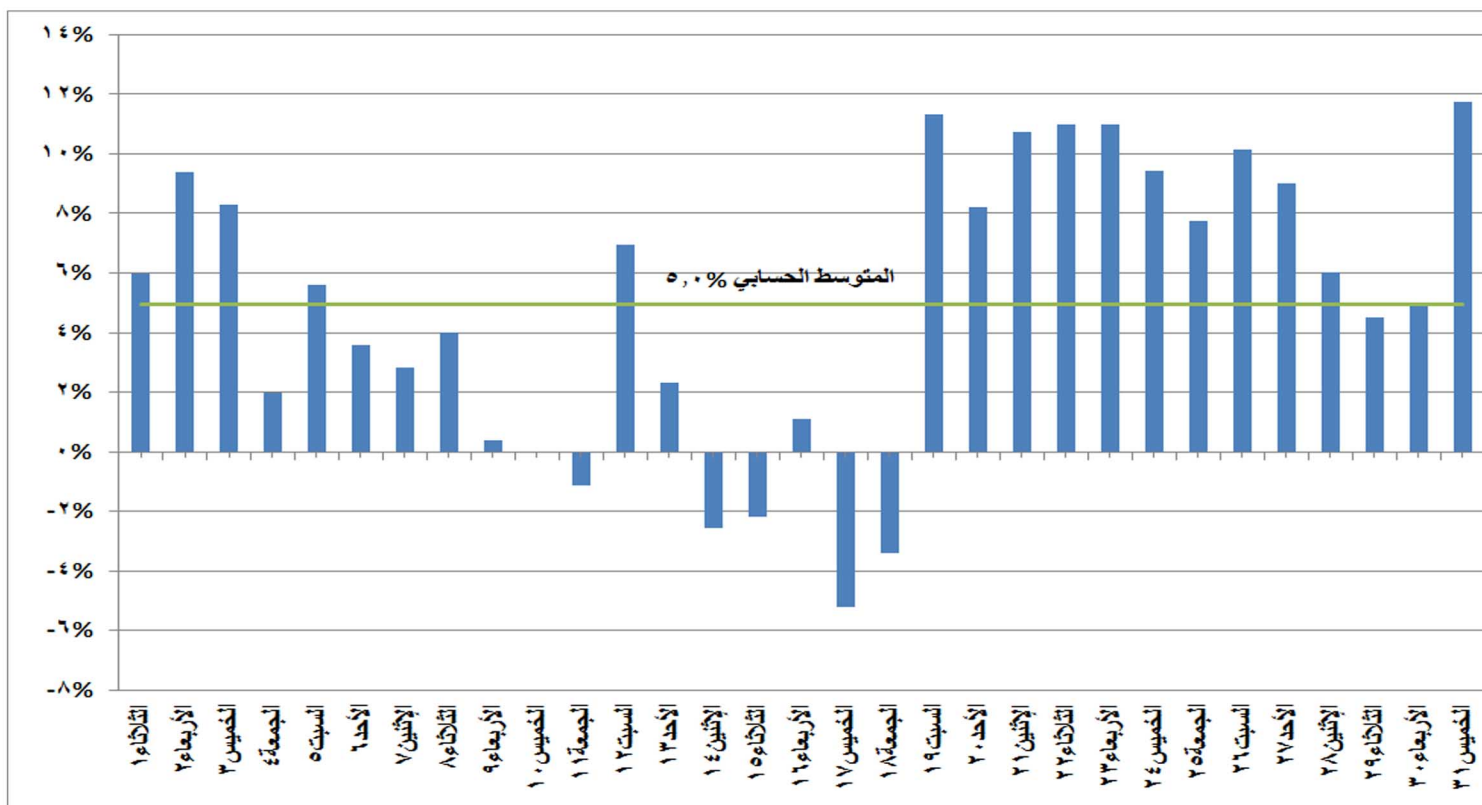
شكل (٩) النسب المئوية للتغير في الحمل الاقصى خلال شهر مايو ٢٠١٨ مقارنة باليوم المماثل من العام الماضي
