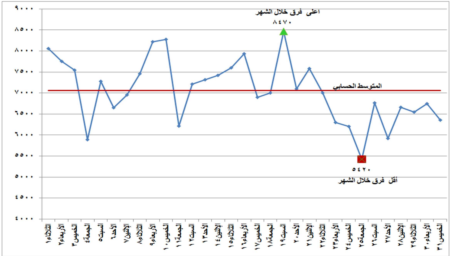
شكل (٣) الفرق بين أقصى وأدنى حمل خلال شهر مايو ٢٠١٨
