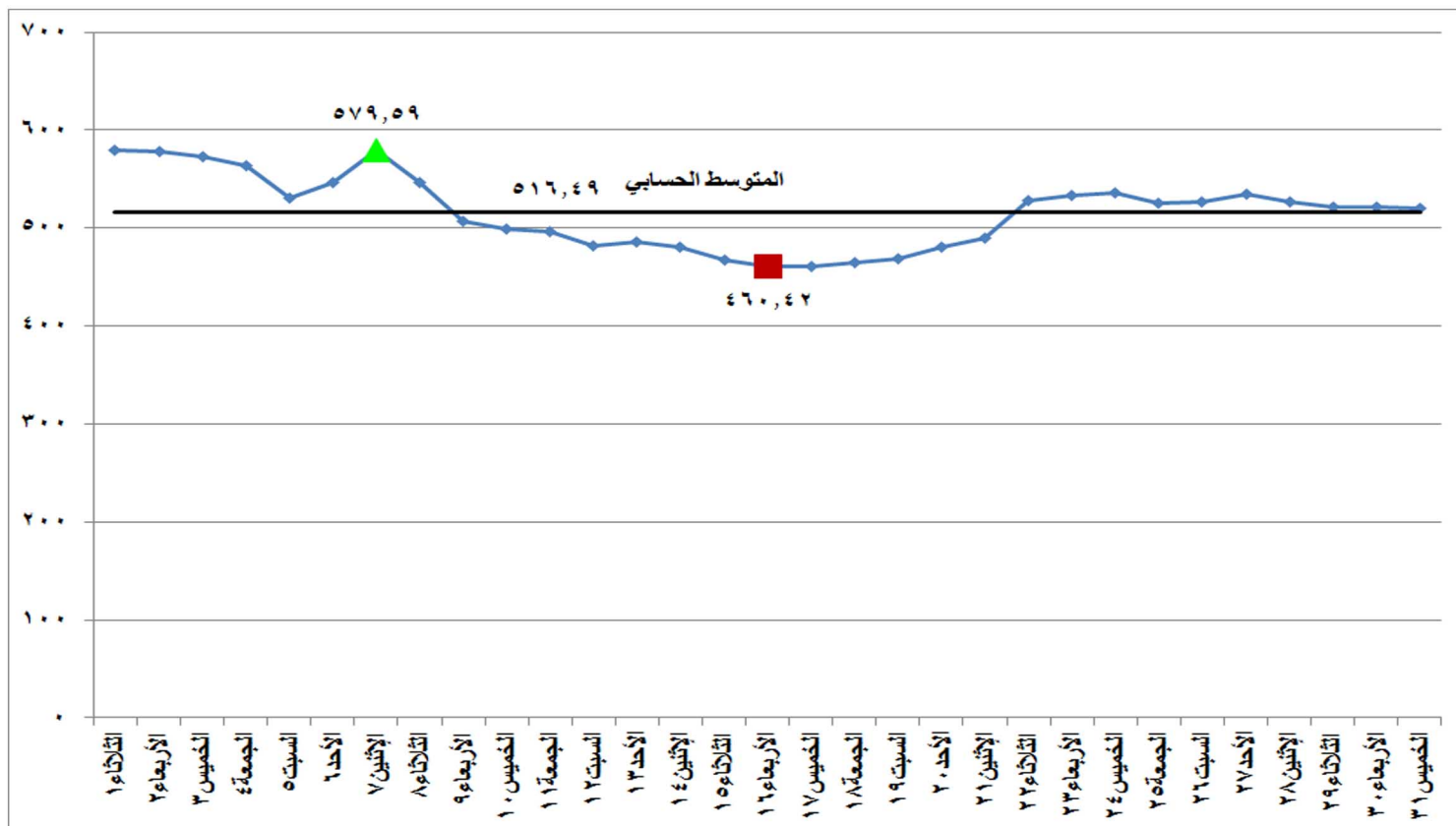
شكل (١٤) معامل انبعاثات غاز ثاني اكسيد الكربون المكافئ على مدى شهر مايو ٢٠١٨
