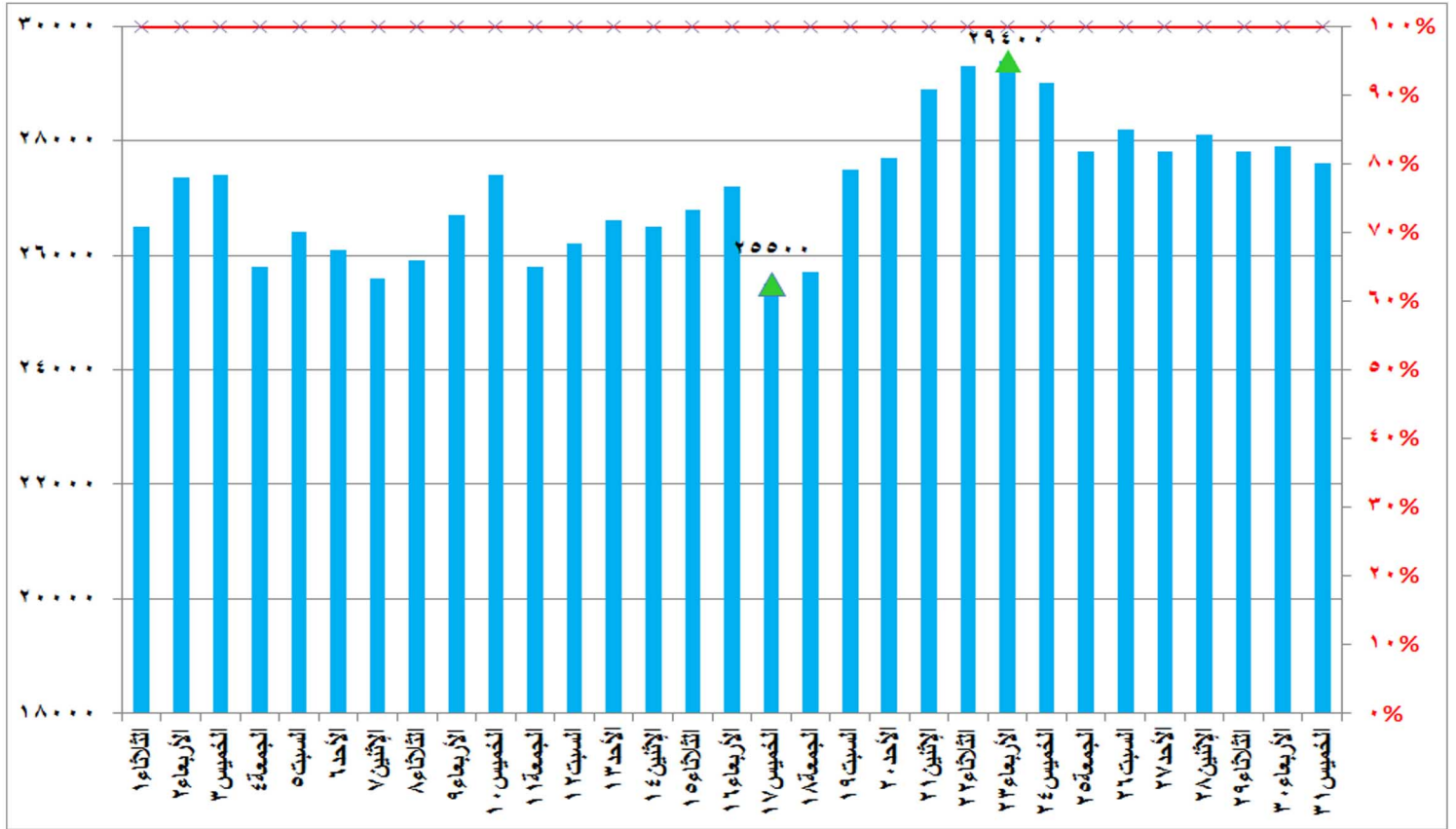
شكل (٥) قدرات الانتاج المتاحة ونسبتها للحمل الأقصى خلال شهر مايو ٢٠١٨
