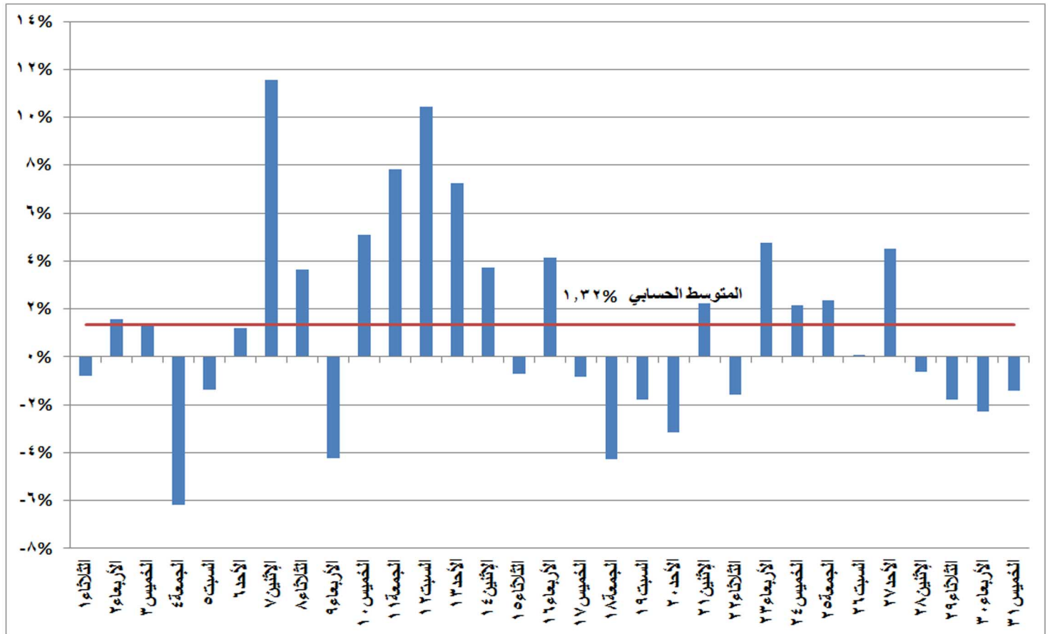
شكل (٢٤) نسب التغير في استخدام المصادر المائية في إنتاج الطاقة الكهربائية خلال شهر مايو ٢٠١٨ مقارنة بالشهر المماثل من العام السابق
