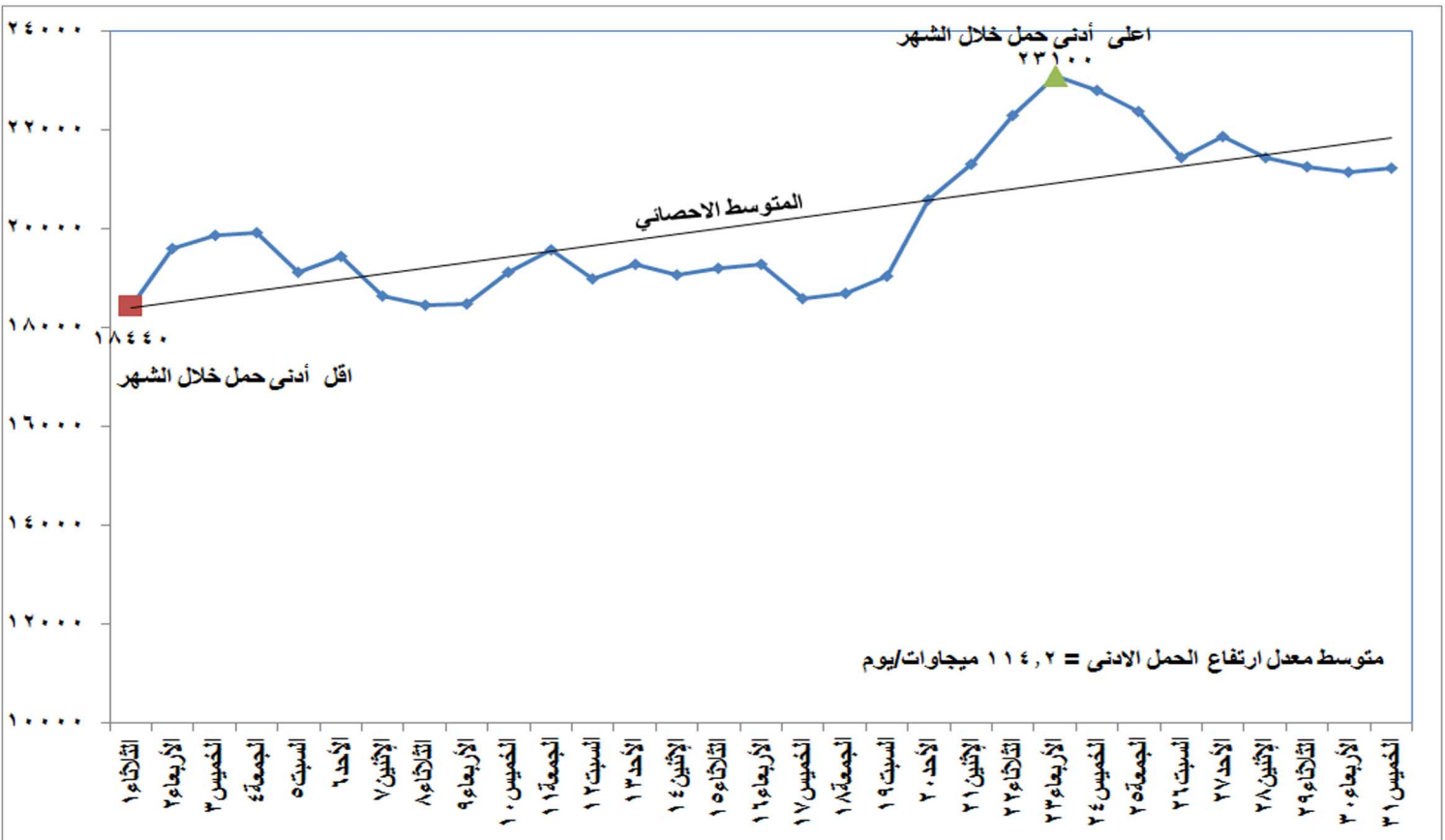
شكل (٢) تطور الحمل الادنى اليومي خلال شهر مايو ٢٠١٨
