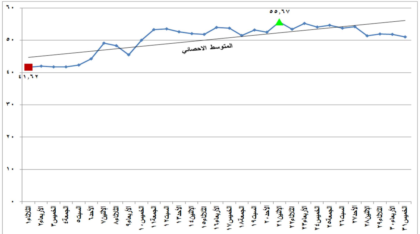
شكل (٢٣) الطاقة الكهربائية المنتجة من المصادر المائية خلال شهر مايو ٢٠١٨
