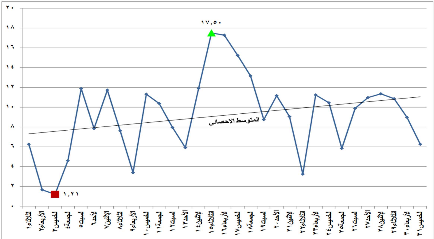
شكل (٢٥) الطاقة الكهربائية المنتجة من الرياح والشمس خلال شهر مايو ٢٠١٨
