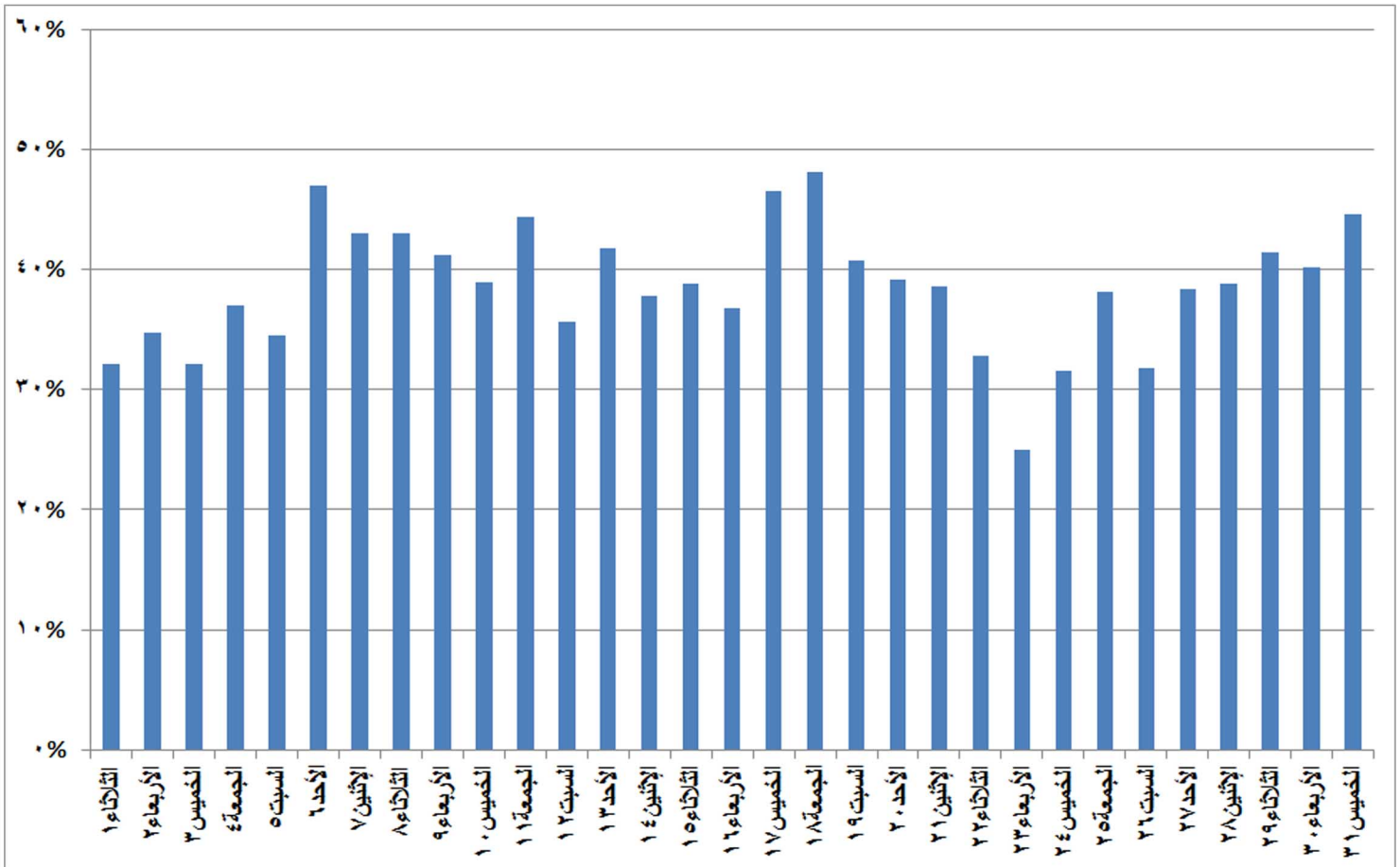
شكل (٢٨) نسب الفائض للحمل الاقصى المسجل يوميا خلال شهر مايو ٢٠١٨
