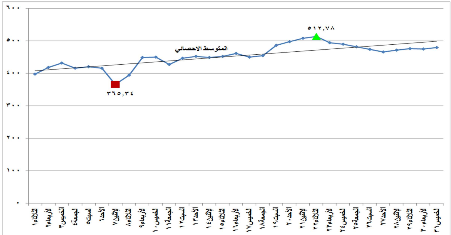
شكل (١٧) الطاقة الكهربائية المنتجة من الغاز الطبيعي خلال شهر مايو ٢٠١٨
