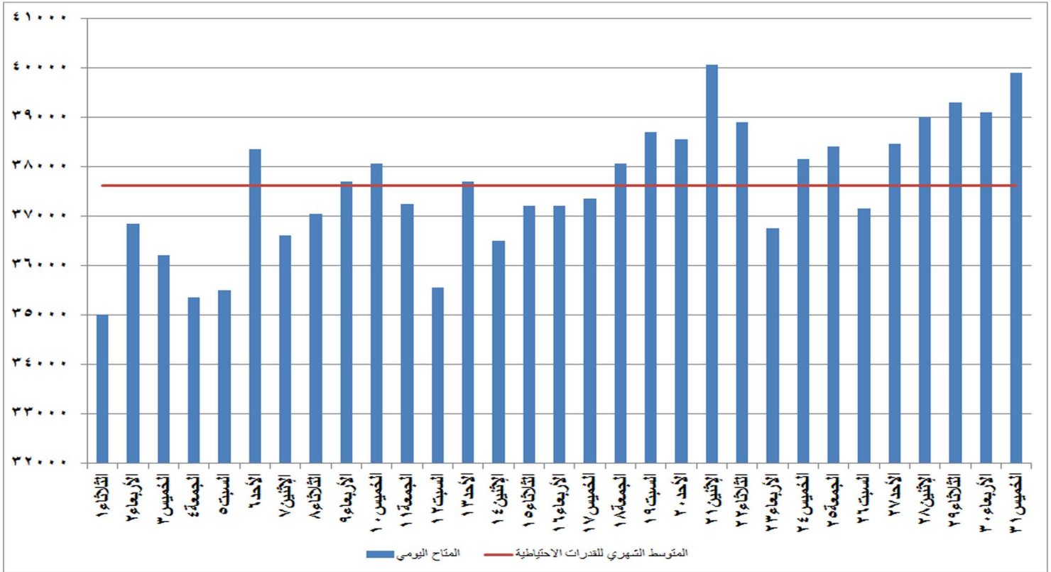
شكل (٢٧) القدرات المتاحة يوميا والمتوسط الشهري للقدرات الاحتياطية خلال شهر مايو ٢٠١٨
