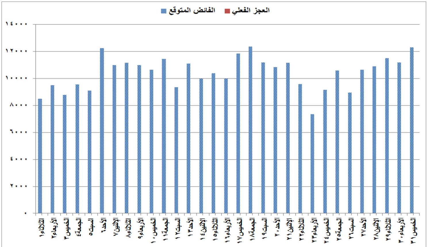
شكل (٧) الفائض والعجز المتوقع للقدرات خلال شهر مايو ٢٠١٨
