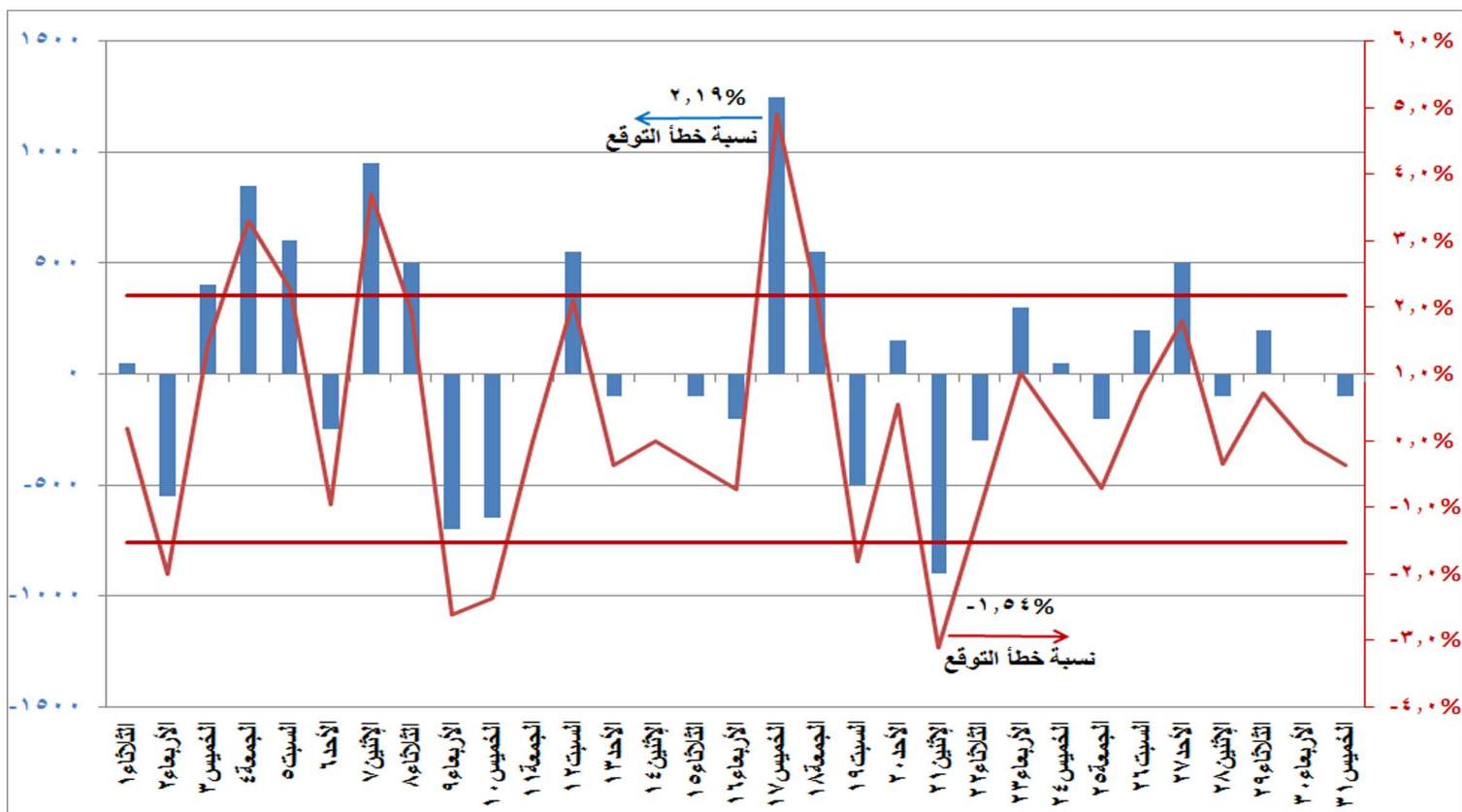
شكل (١٠) الفرق بين الحمل الأقصى المتوقع والمسجل فعليا ونسبة الفرق إلى الحمل المسجل فعليا خلال شهر مايو ٢٠١٨
